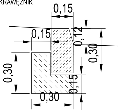
2.KRAWĘŻNIK WTOPIONY
