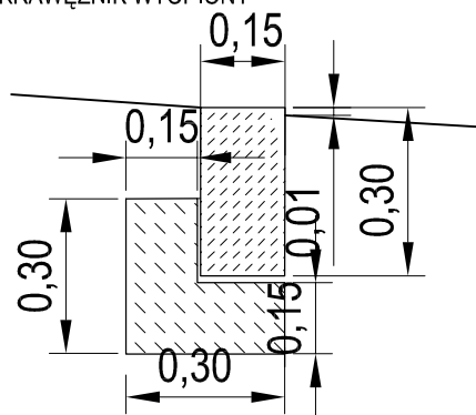
2.KRAWĘŻNIK WTOPIONY
