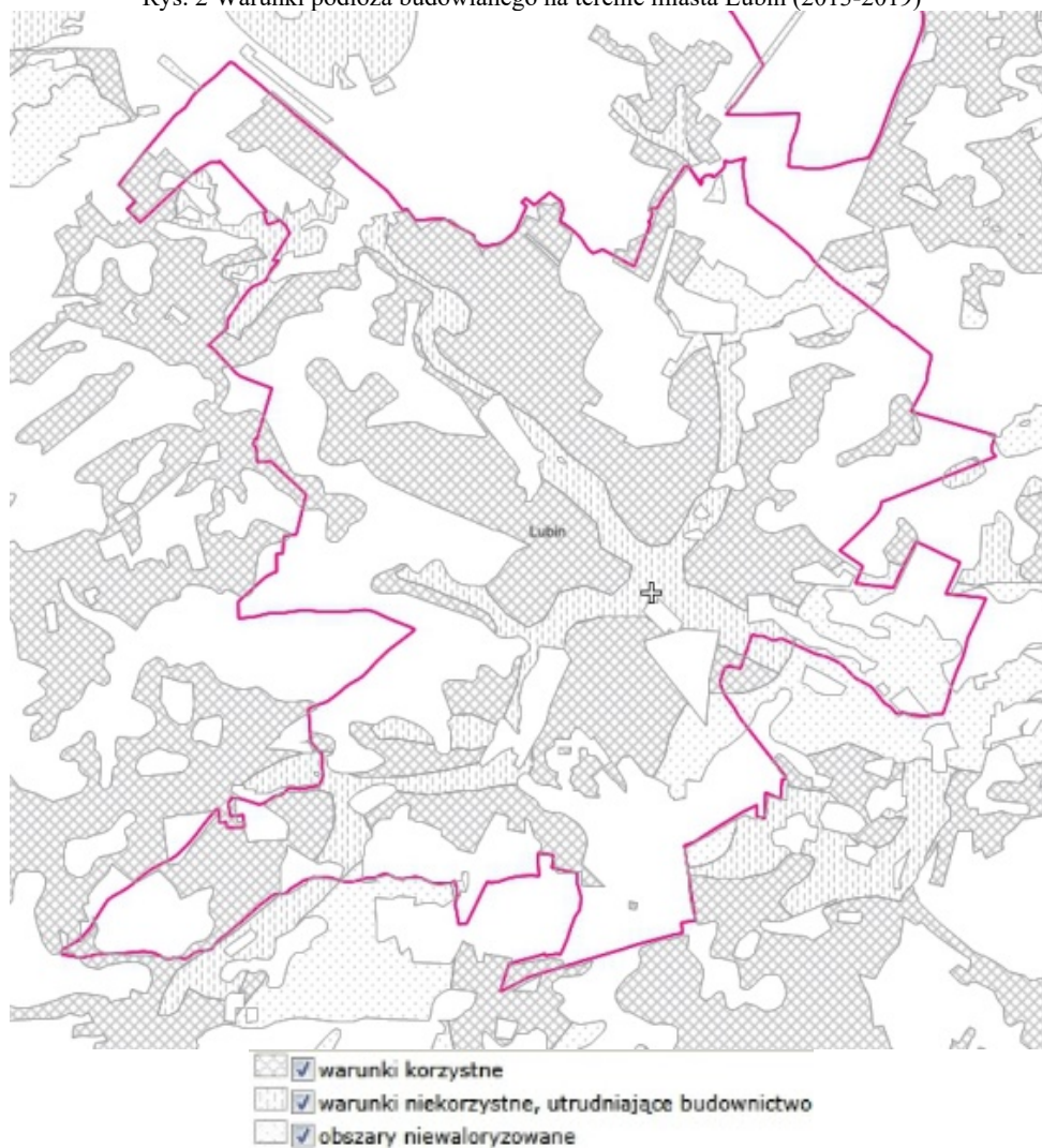
Rys. 2 Warunki podłoża budowlanego na terenie miasta Lubin (2013-2019)
