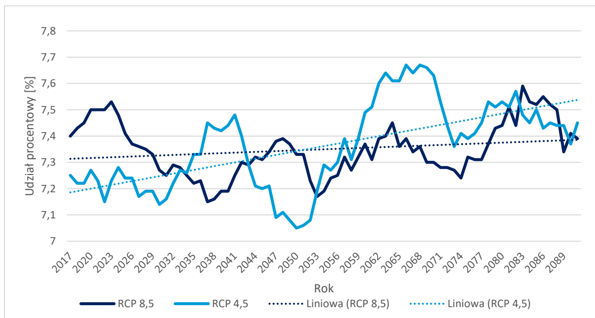
Wykres 26. Prognoza dotycząca średniej kroczącej średniego udziału ciszy (< 1 m/s) - powiat lubiński 97
