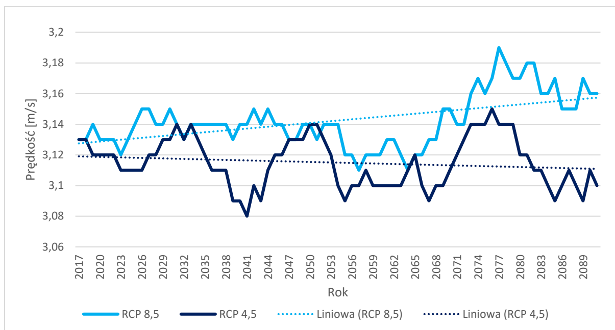
Wykres 25. Scenariusz RCP 4,5 oraz RCP 8,5. Prognoza dotycząca średniej miesięcznej prędkości wiatru - powiat lubiński 96
